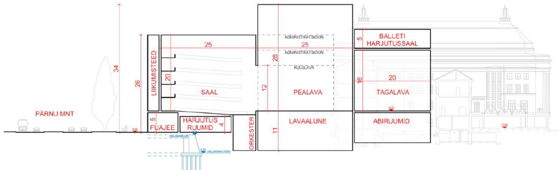
LÕIGE A-A
